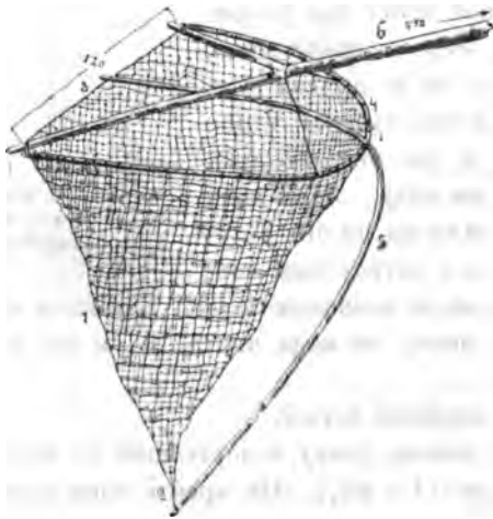
147. Сак. 1. саківно; 2. готовник; 3. попруга; 4. дуга; 5. облук; 6. держак з вилами, до яких прислана дуга поворозом до держака.
