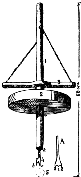
196. Друлівник. 1. било; 2. кочало; 3. валок; 4. писачок; а. шпиль; б. околичник; с. сердешник. А писачок з двома околичниками (2) і сердешником (1).
