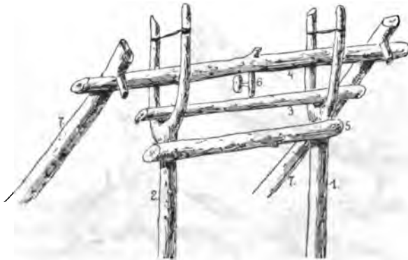
161. Підколовда. 1, 2. Сохи з лубом; 3. підколовдина; 4. круглий притяг; 5. победрина; 6. свердлик з фостиком, на кінці мясо; 7, 7. тижкі пільги, які опирають ся на притягу; верх пільг накладають лат і фої.
