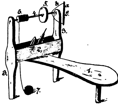
177. Ремісник. 1. сідєц; 2. скринка; 3. 3. лаби; 4. веретєно; 5. колєсо; 6. цівка; 7. клубок; 8. лучок а. ручка , б. ремєнєц . В скринці (2): човник, веретєно, клубок.
