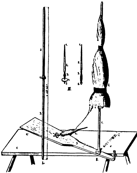
94. I. Кужівка . 1. кочало; 2. кужівник; 3. держівно. II. Кужівка (1) з кужїлем (2) затинена у сїдець (3); 4. простень. III. Веретено . 1. спїнь; 2. череве; 3. затинка; 4. кочальце; б. гуска.
